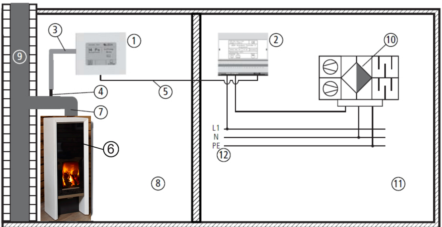
Schema Einbau- und Installation LUC
